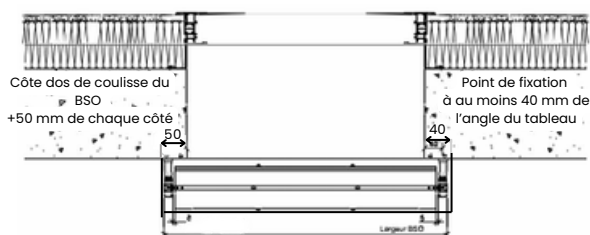
BSO POSE EN APPLIQUE SUR LA FAÇADE — LAMBREQUIN TYPE 8
