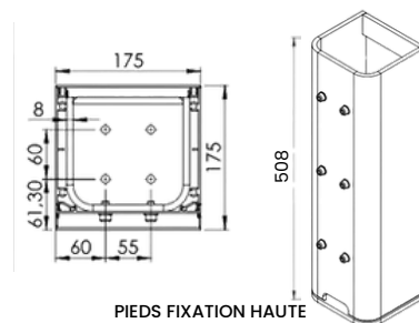
PIEDS FIXATION HAUTE
