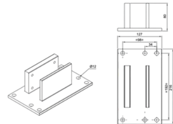
PLATINES DE FIXATION
