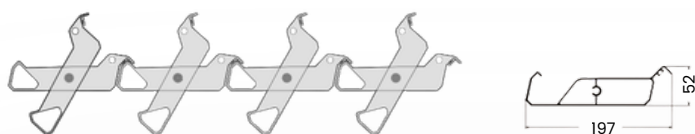
LAME DOUBLE PAROI
