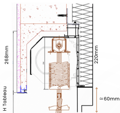
MAISON OSSATURE BOIS
