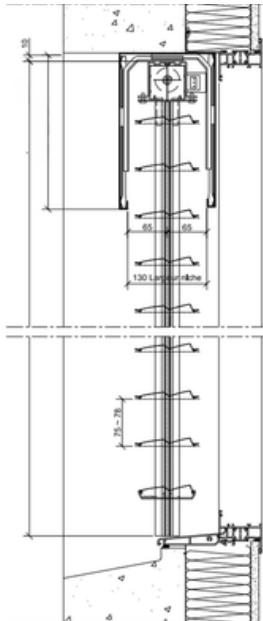
POSE DE FACE LAMBREQUIN TYPE 9
