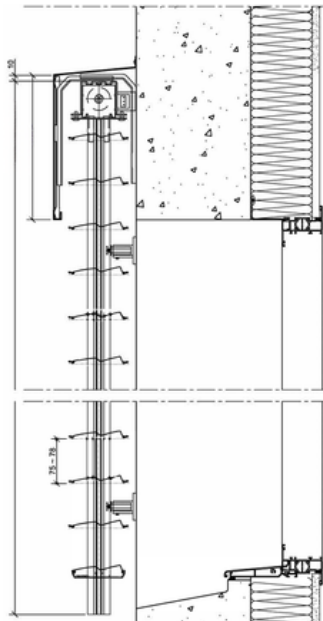
POSE EN APPLIQUE SUR LA FAÇADE LAMBREQUIN TYPE 8
