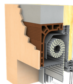
DEMI LINTEAU MAÇONNERIE Enroulement maxi ø160
