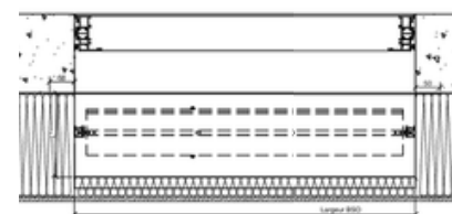
BSO POSE DANS ITE AVEC LAMBREQUIN ITE
