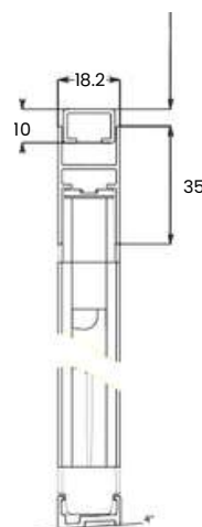
PROFIL LATÉRAL
