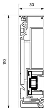
COULISSE VP110 VISIBLE/CACHÉE
