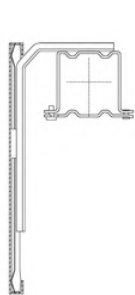
LAMBREQUINS TYPE 1
