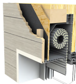
MAISON OSSATURE BOIS Enroulement maxi ø200
