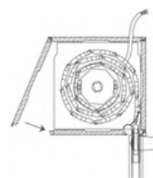
Trappe de visite coté intérieur
