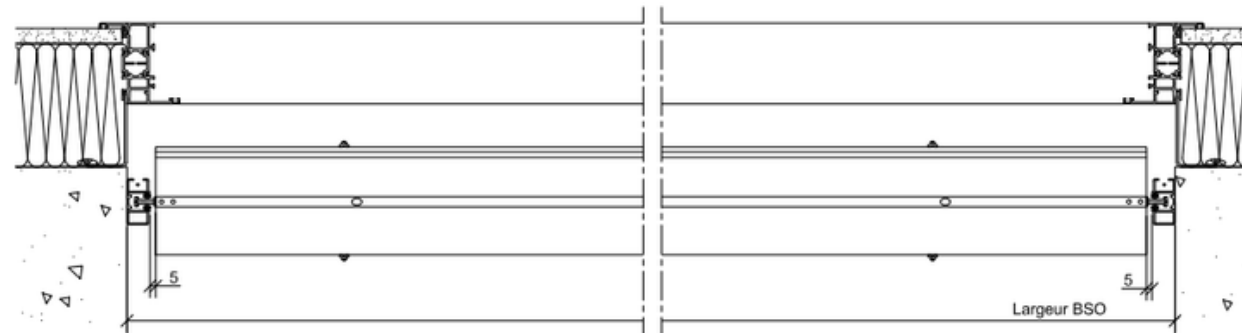
Coupe horizontale Z-Line 90 Coulisse auto-portée Lambrequin type 9
