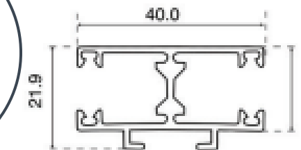
DPF Coulisse double pose de face
