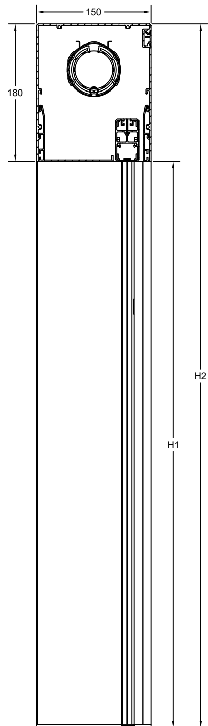
Coupe A-A
