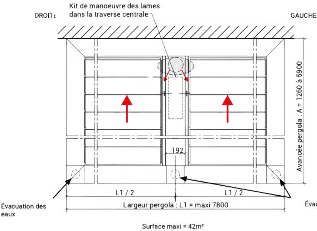
2 modules lames parallèles à la façade avec poteau intermédiaire
