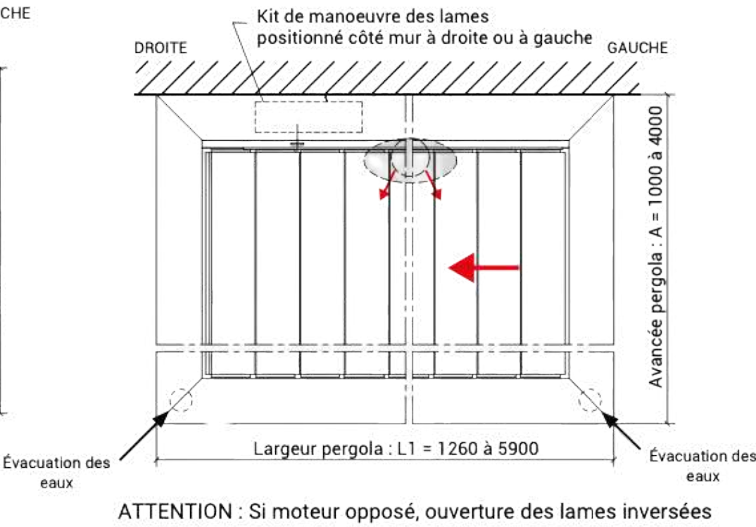
1 module lames perpendiculaires à la façade
