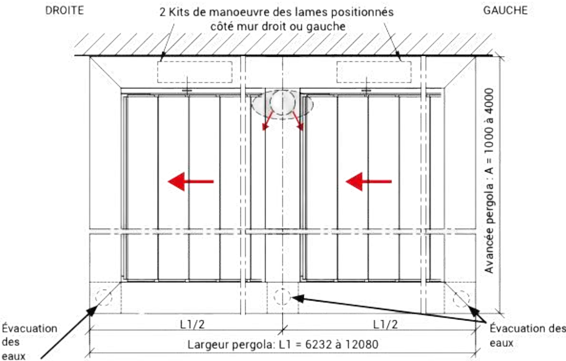
2 modules lames perpendiculaires à la façade avec poteau intermédiaire
