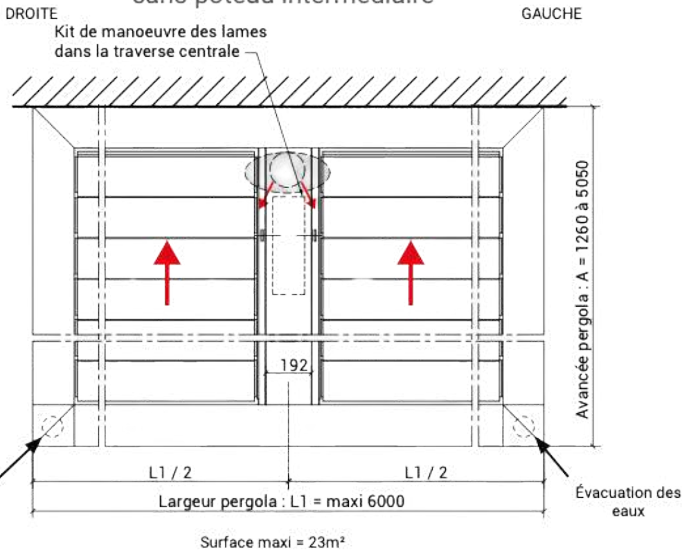
2 modules lames parallèles à la façade sans poteau intermédiaire
