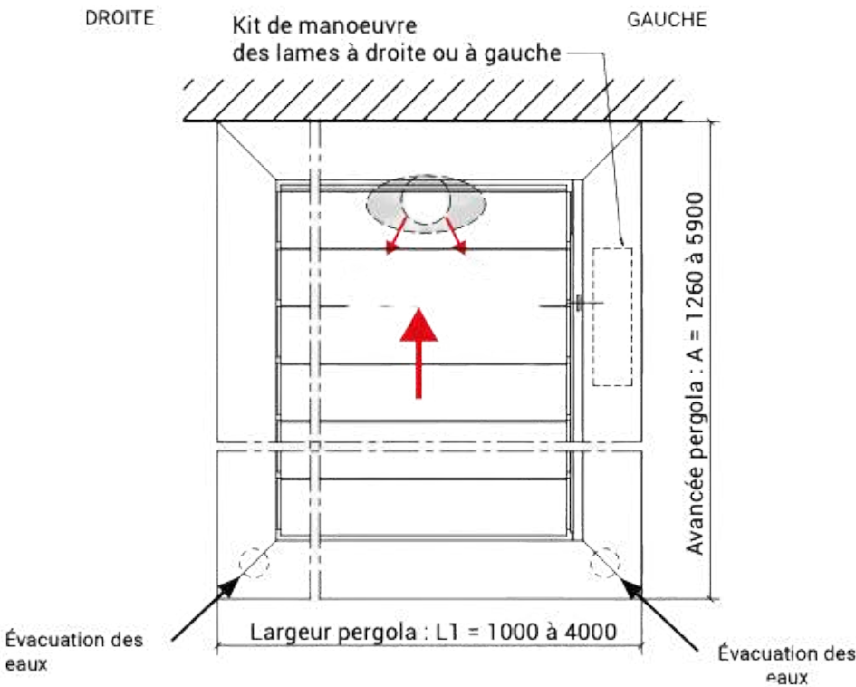
2 modules lames parallèles à la façade avec poteau intermédiaire
