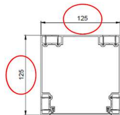
Poteau avec capot droit
