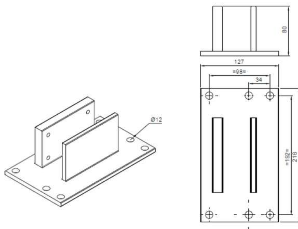
Platine de fixation
