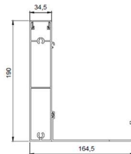
Poutre avec chéneau
