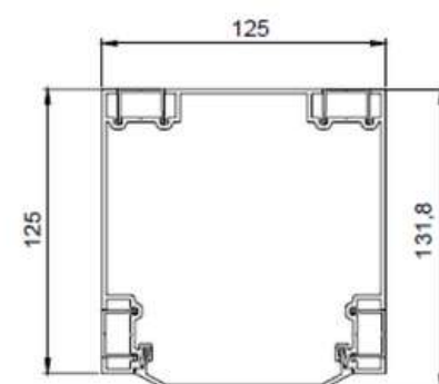
Poteau avec capot chanfreiné (option)
