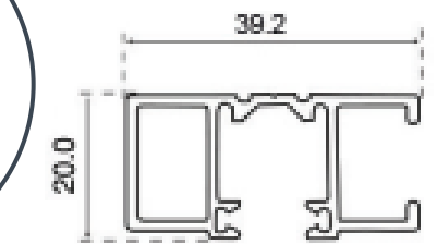
AP Coulisse autoportée
