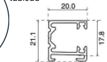
SFP Coulisse simple pose de face et pose tableau
