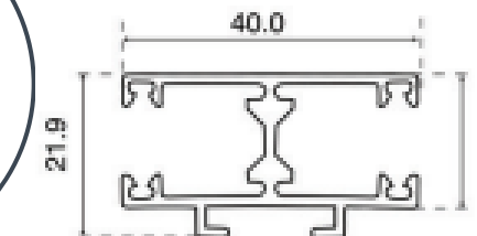
DPF Coulisse double pose de face
