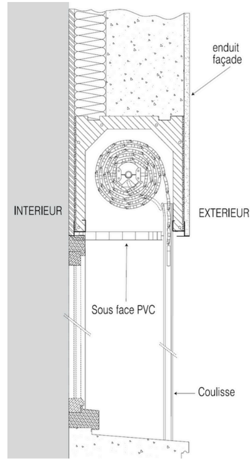
COFFRE CLM 28 VOLET ENROULEMENT INTÉRIEUR
