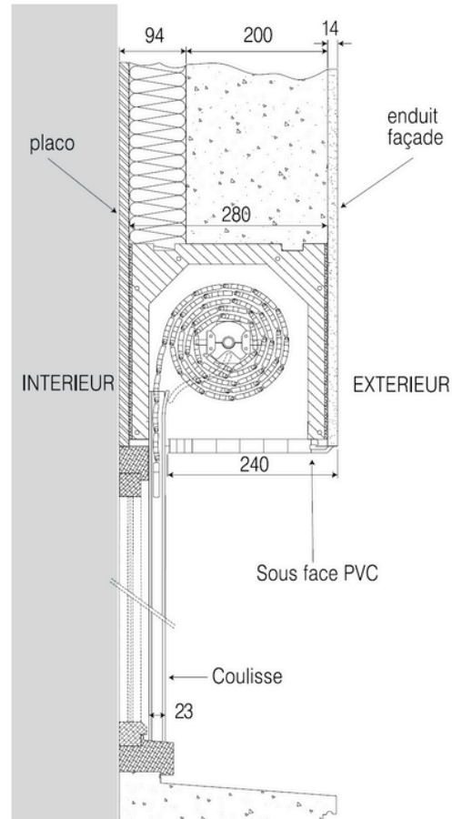
COFFRE CLM 28 SORTIE ÉLECTRIQUE / ENROULEMENT EXTÉRIEUR
