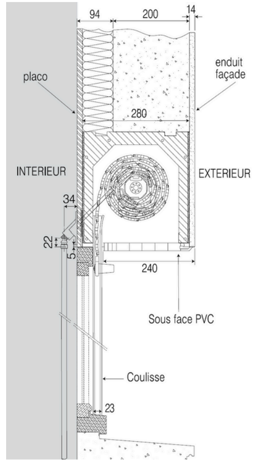
COFFRE CLM 28 SORTIE TREUIL / ENROULEMENT EXTÉRIEUR
