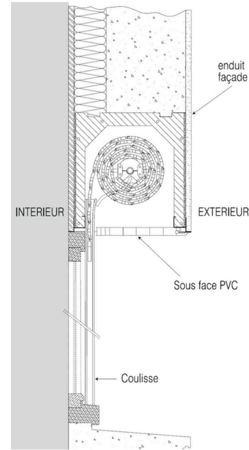
COFFRE CLM 28 VOLET ENROULEMENT EXTÉRIEUR
