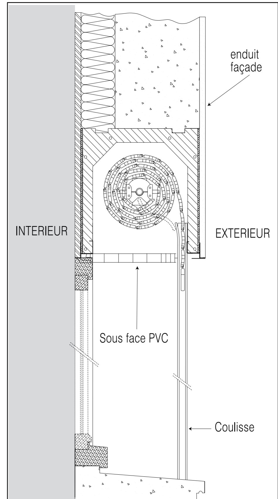
COFFRE CLM 28 VOLET ENROULEMENT INTÉRIEUR
