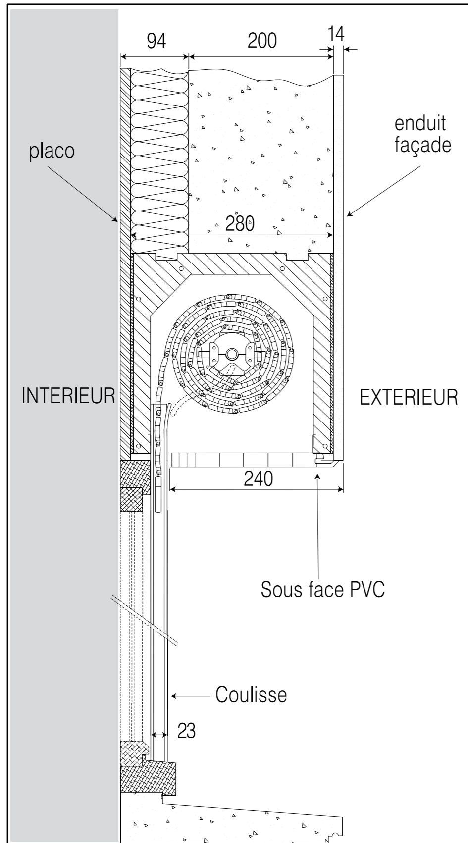
COFFRE CLM 28 SORTIE ÉLECTRIQUE / ENROULEMENT EXTÉRIEUR
